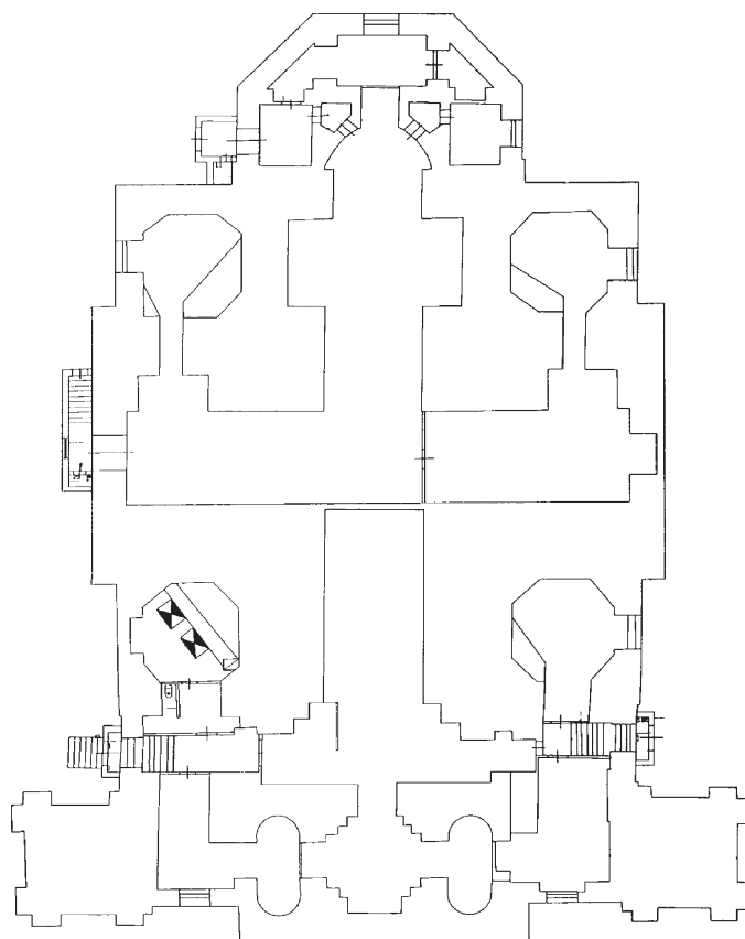
План криптового этажа Екатерининского собора г. Краснодара. Состояние на 2018 г.
