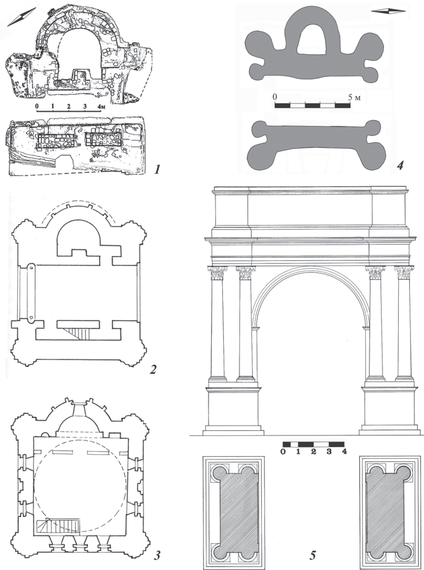
Рис. 4. Аналоги к реконструкции сооружения по ул. Владимирской, № 3: 1–3 – ворота с надвратной церковью Михайловского монастыря (1 – план, 2–3 – реконструкция верхнего и нижнего ярусов); 4 – реконструкция планировки фундаментов постройки по ул. Владимирской, № 3; 5 – арка II в. до н. э., Коринф.
