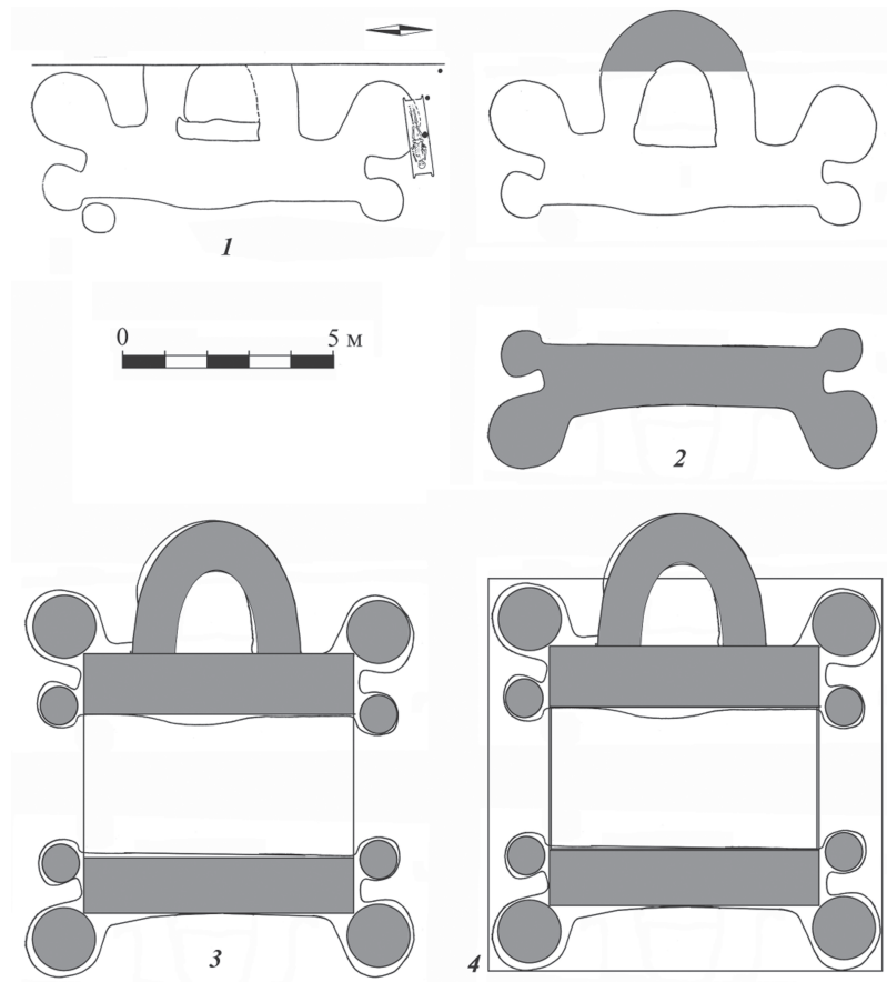
Рис. 3. Постройка по ул. Владимирской, № 3. Реконструкция фундаментов и стен, предложенная А. В. Комаром. См.: Комар О. В. «Дохристиянська» монументальна архітектура Старокиївської гори (проблеми датування та атрибуції) // Opus Mixtum. 2013. № 1. С. 110.
